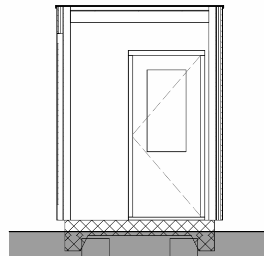
doorsnede
